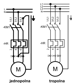
Šema veze
